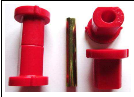
Artikel-Nr: 110127 PU-Blattfederbuchsen VA außen f. Sportblattfeder
